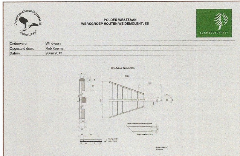
Een werktekening van de windvaan, gemaakt door Rob Koeman
